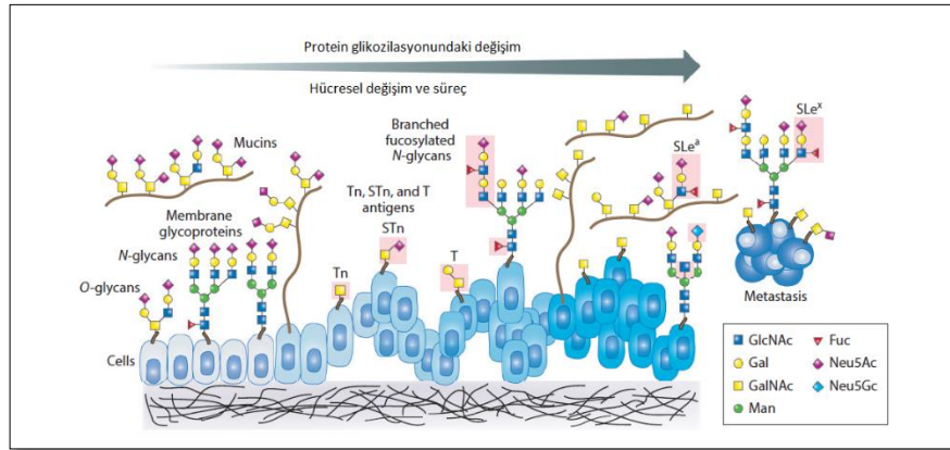
Şekil 2.11. Protein glikozilasyonu boyunca değişimler. Tn, STn, T antijenleri oluşumu, fukoziilasylanmış zincirler ve metastaz. Kırmızı kutucuk içerisinde alınmış moleküller kanser belirtilerini temsil etmektedir [22].
