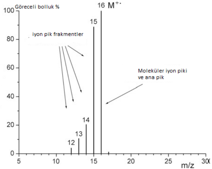
Şekil 2.16. Düşük kütleli hidrokarbonun elektrik iyonizasyon kütle spekturumu [30].
