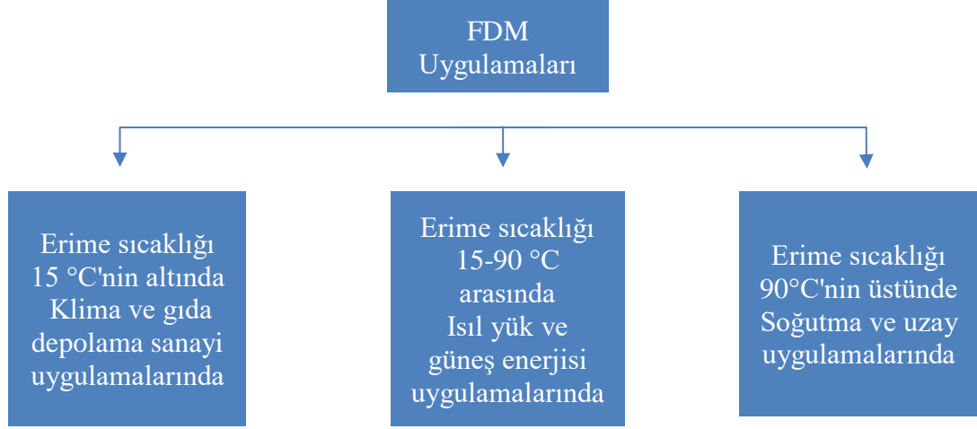
Şekil 3.4. Erime sıcaklığına göre FDM'lerin sınıflandırılması
