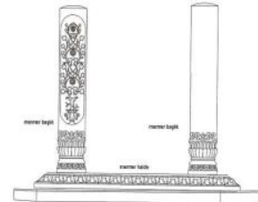
ARKA GÖRÜNÜŞ
