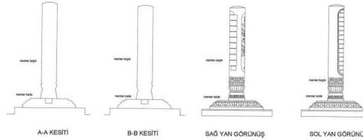
A-A KESİTİ
