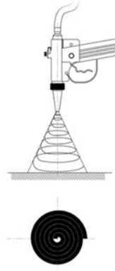
Şekil 2.29. Mikro kumlama yönteminde granüllerin yüzeye dairesel hareketle yaklaşması ve hafif temaslarla temizliği (İnternet, 9).
