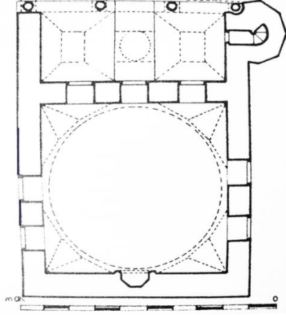
Şekil 4.18. Alaaddin Bey Camii planı (Kaplanoğlu, 1994).
