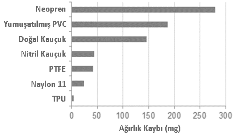
Şekil 2.3. Bazı endüstriyel malzemelerin aşınma dirençlerinin kıyası [9].
