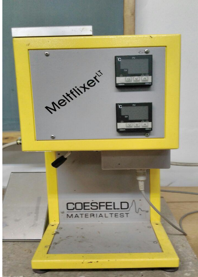
Şekil 5.11. Meltfixer LT marka erime akış indeksi ölçüm cihazı.
