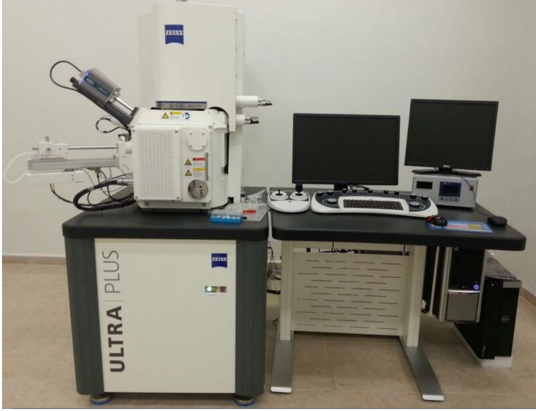
Şekil 5.7. Carl Zeiss Ultra Plus Gemini taramalı elektron mikroskobu [36].
