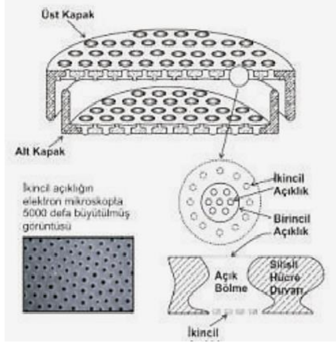
Şekil 3.3. Elips şekilli bir diatomitin yapısının tasviri [11].
