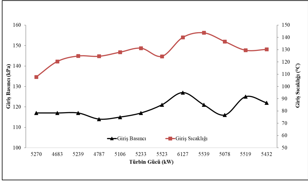
Şekil 5.2. Giriş basıncı ve sıcaklığa göre türbin gücündeki değişim.
