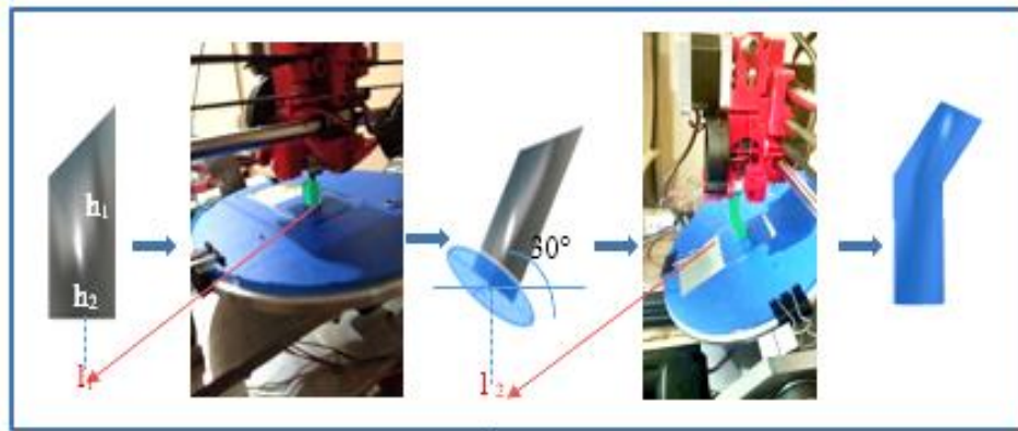
Şekil 5.13. 5 eksen yazdırma aşamaları.
