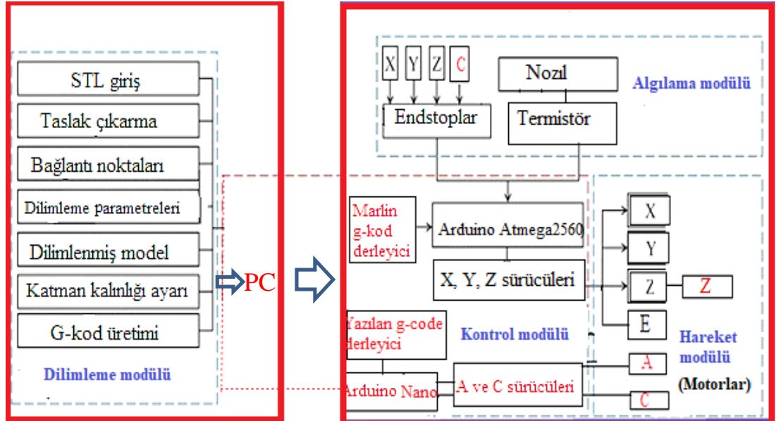
Şekil 5.1. 5 Eksen 3B yazıcının kontrol ünitesi.
