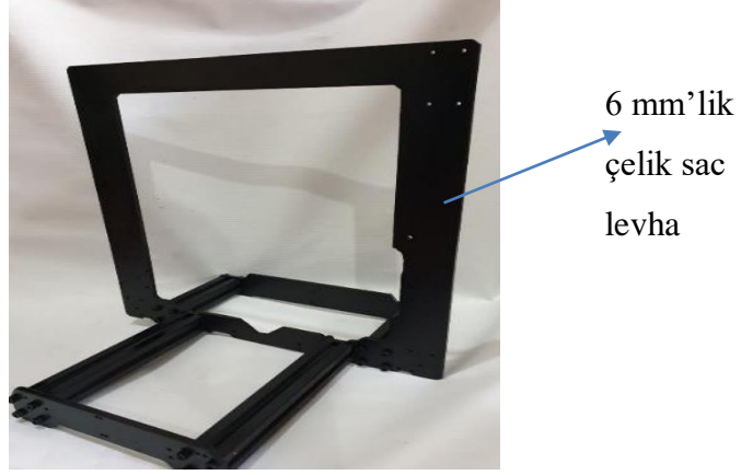
Şekil 4.3. 5 eksen 3B yazıcı çelik sactan imal edilen gövde.
