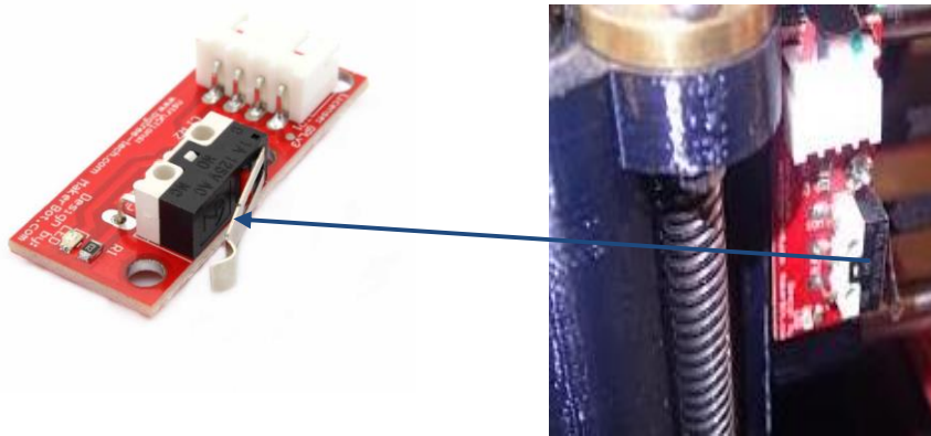
Şekil 5.8. Endstop.
