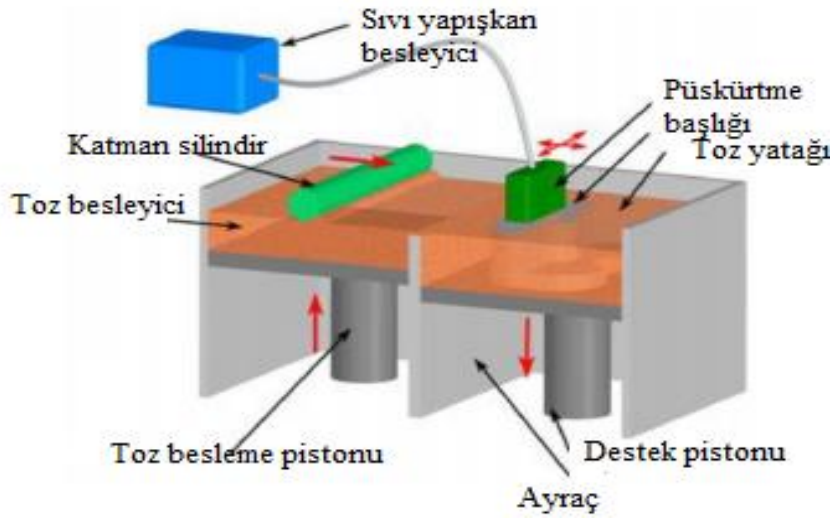
Şekil.3.6. Binder jet teknolojisi [45].
