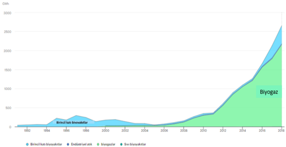
Şekil 3.42. Kaynaklarına göre biyoyakıt ve atıklardan elektrik üretiminin 1991-2018 yılı aralığındaki değişimi [30].
