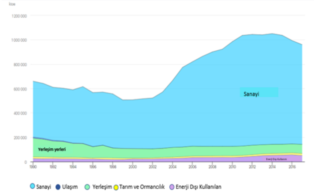
Şekil 3.7.Dünyada sektörlere göre kömür tüketimi [28].
