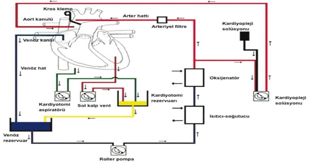
Şekil 1. Standart bir KPB düzeneği.
